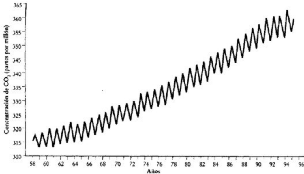
Concentraciones de dióxido de carbono en la atmósfera terrestre a lo largo del tiempo
